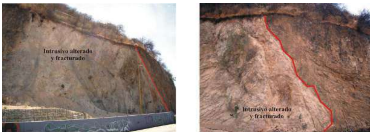
Figura 5.3.12. Afloramiento de la roca granítica alterada sobre el trazo de la carretera del cerro El Fortín. La fotografía de la derecha es un acercamiento del mismo punto.
