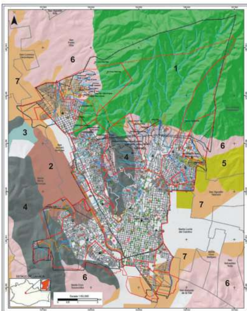
Figura 3.14. Mapa edafológico del municipio de Oaxaca de Juárez. 1: Acrisol. 2: Feozem. 3: Fluvisol. 4: Litosol. 5: Luvisol. 6: Regosol. 7: Vertisol. Fuente: Mapa de Suelos, INEGI serie I, escala 1:250,000.
