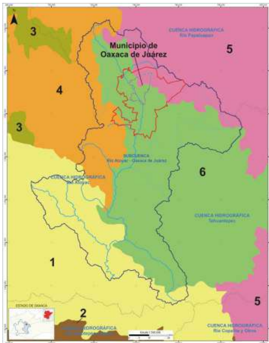
Figura 3.2 Subprovincias fisiográficas y cuencas hidrográficas de la zona central del estado de Oaxaca. 1: Cordillera Costera del Sur, 2: Costas del Sur, 3: Mixteca Alta, 4: Sierras Centrales de Oaxaca, 5: Sierras Orientales, 6: Sierras y Valles de Oaxaca. La línea roja indica el límite de la zona metropolitana de Oaxaca. Modificado de: Red hidrográfica SIATL, INEGI, y Subprovincias fisiográficas, INEGI, escala 1:1000,000.
