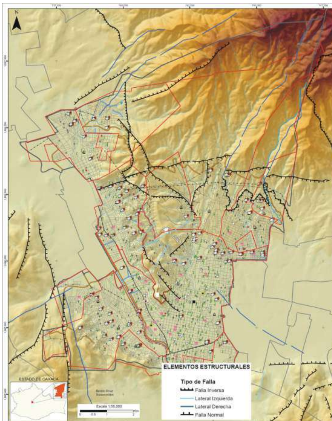
Figura 5.1.1. Mapa que muestra los principales sistemas de fallas y fracturas dentro del área de estudio.
