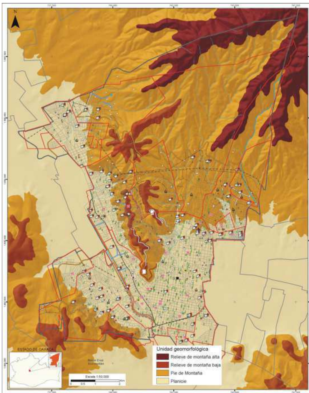
Figura 3.13. Mapa con las principales unidades geomorfológicas de la zona de estudio.
