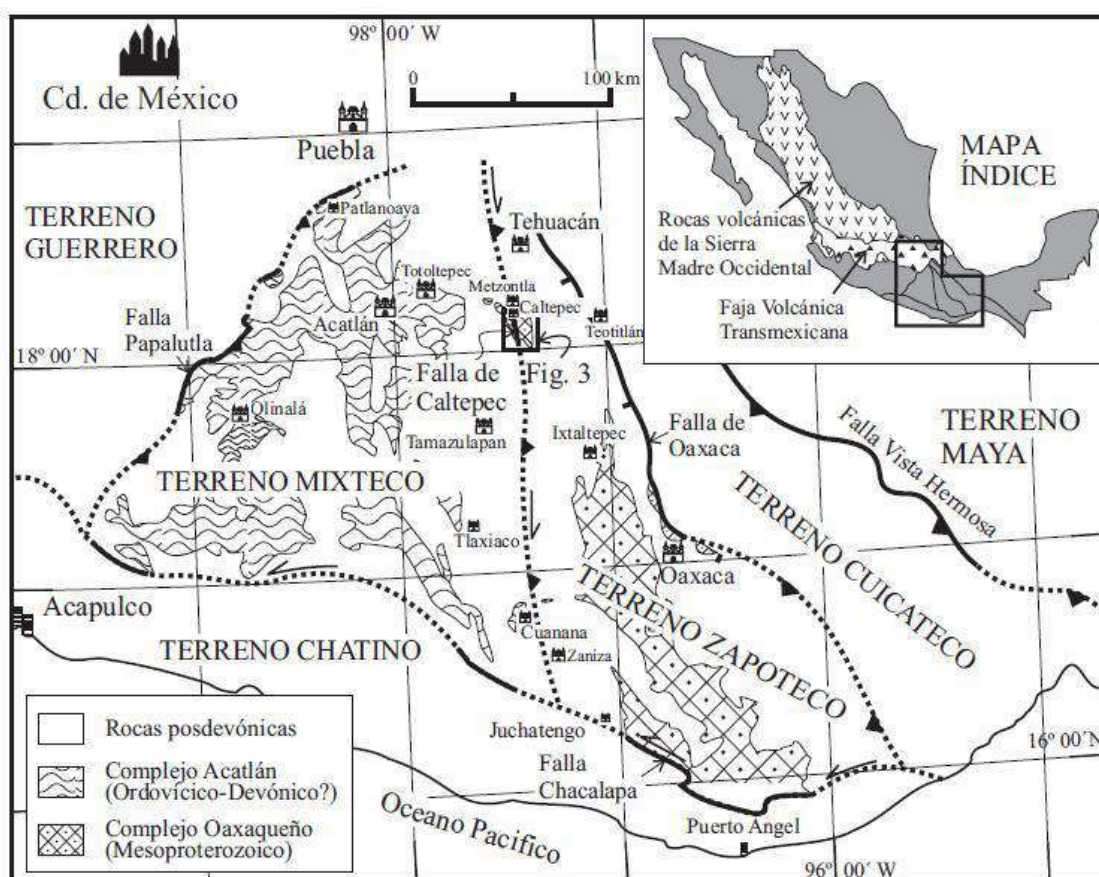
Figura 3.3. Mapa que muestra la distribución de los terrenos tectónicos del sur de México y las fallas que los limitan. Fuente: Elías-Herrera et al. , 2005.
