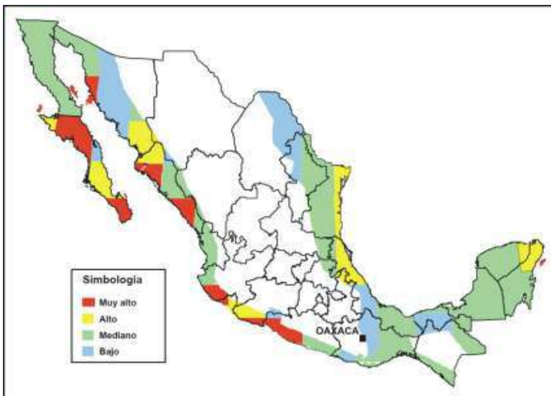
Figura 1.5. Mapa de presencia de ciclones tropicales en la República Mexicana. Fuente: CENAPRED ( http://www.cenapred.gob.mx/es/Investigacion/RHidrometeorologicos/FenomenosMeteorologicos/CiclonesTropicales ).
