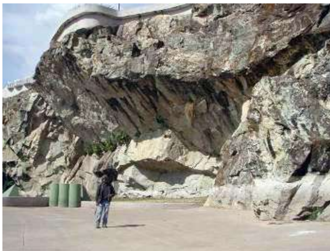
Figura 3.11. Ignimbrita color verde claro en un corte en el parque Las Canteras.
