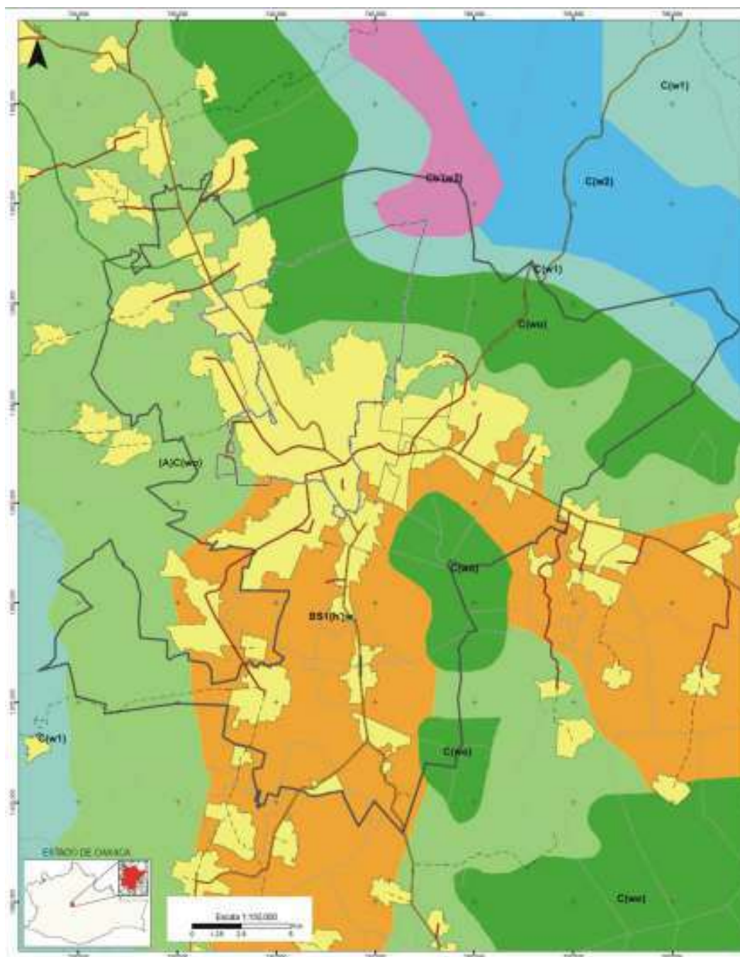
Figura 3.18. Mapa con la distribución de los diferentes tipos de climas que predominan en la zona de estudio. AC(w0): semicálido-subhúmedo, (Cb)w2: semifrío, BS1(h')w: semiárido cálido y tres tipos de templado subhúmedo C(w1), C(w)2 y C(w0). Los polígonos en amarillo delimitan áreas urbanas. El polígono en línea oscura delimita la zona metropolitana de Oaxaca. Fuente INEGI y García, E.-CONABIO, 1998.
