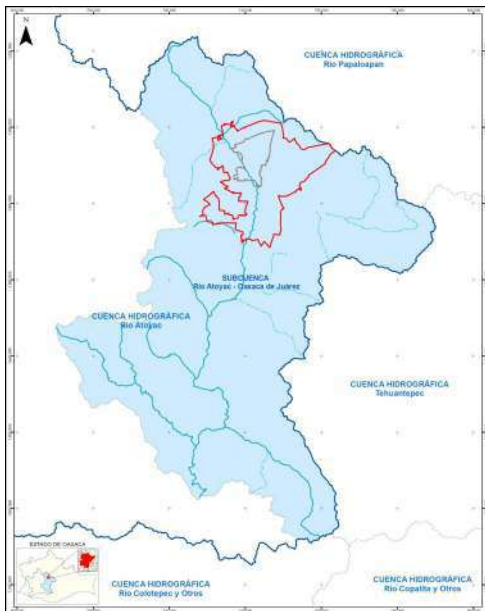
Figura 3.16. Principales cuencas hidrográficas de la región central de Oaxaca. La línea gruesa en azul delimita la región hidrológica Costa Chica-Río Verde, dentro de la cual se encuentra la zona de estudio. Los polígonos con línea roja y gris delimitan la zona metropolitana y el municipio de Oaxaca de Juárez, respectivamente. Fuente: Red Hidrográfica SIATL, INEGI.
