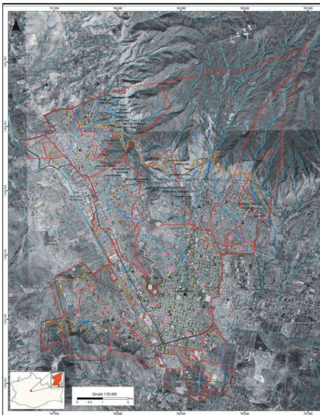
Figura 3.17. Mapa con la red hidrológica de la zona del municipio de Oaxaca de Juárez y áreas circunvecinas.
