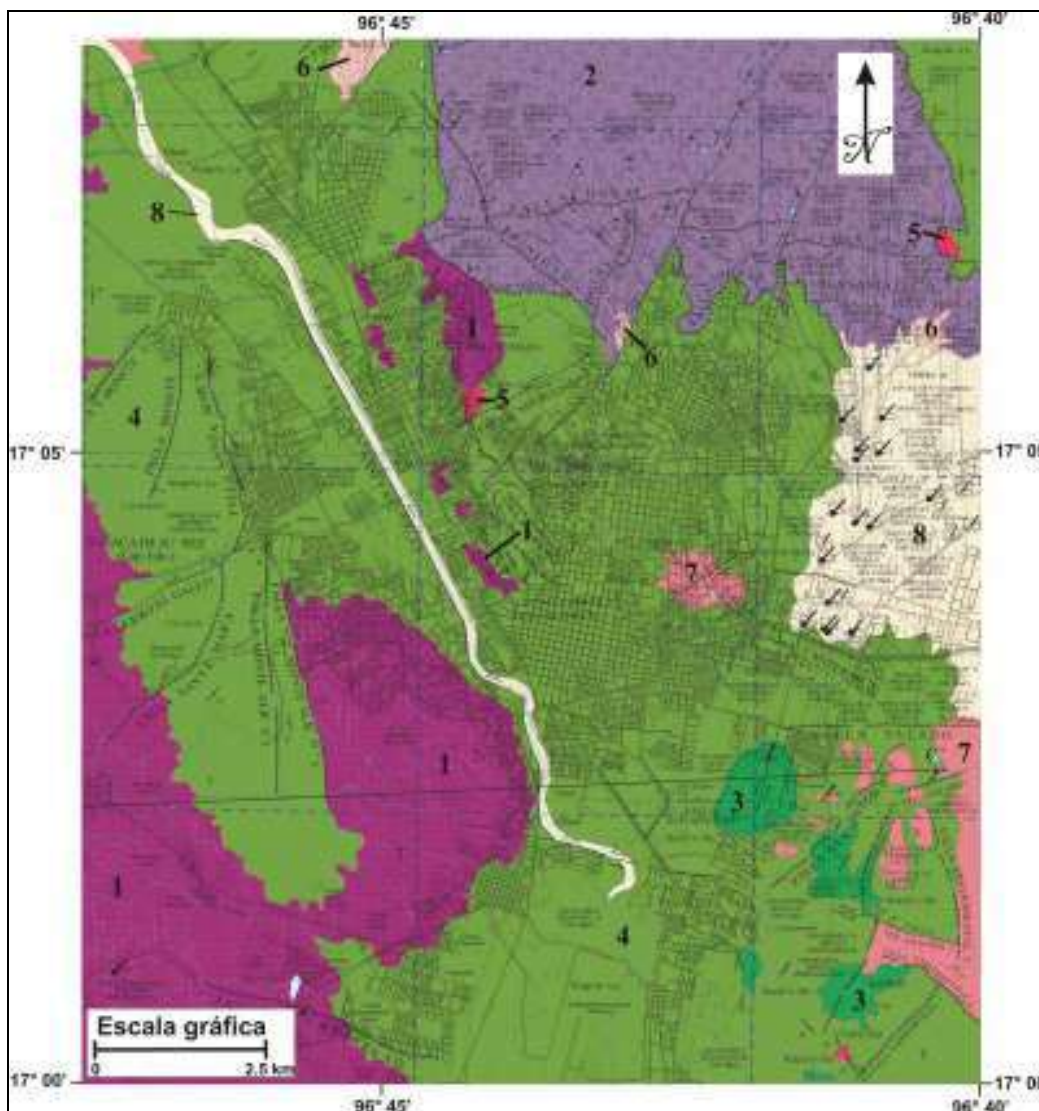
Figura 3.4. Mapa geológico de la zona metropolitana de la ciudad de Oaxaca. 1: Rocas metamórficas del Complejo Oaxaqueño. 2: Rocas de bajo metamorfismo y sedimentarias del Jurásico (Complejo milonítico). 3: Calizas y dolomías del Cretácico. 4: Areniscas y lutitas del Cretácico. 5: Intrusivo granítico del Terciario. 6: Andesita del Terciario. 7: Ignimbrita-conglomerado, toba riolítica del Terciario. 8: Limolita-arena y aluvión del Cuaternario. Modificado de la Carta Geológico-Minera Oaxaca de Juárez (E14-D47), Servicio Geológico Mexicano (2007).
