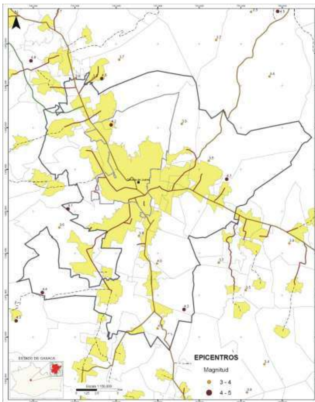
Figura 5.1.2. Mapa con la localización de los epicentros de temblores dentro de la zona metropolitana de Oaxaca y sus alrededores.
