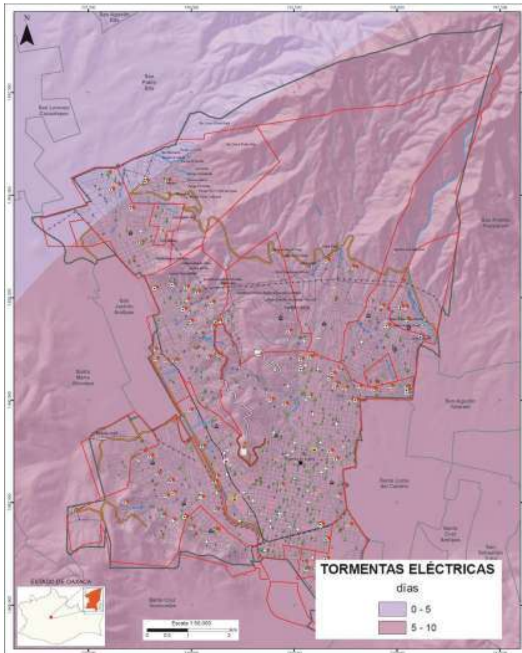
Figura 5.2.2. Días de ocurrencia de tormentas eléctricas dentro del municipio de Oaxaca de Juárez. Fuente: Datos vectoriales INEGI escala 1:50,000, carta E14D47. Normales Climatológicas SMN, periodo de datos 1971-2000.
