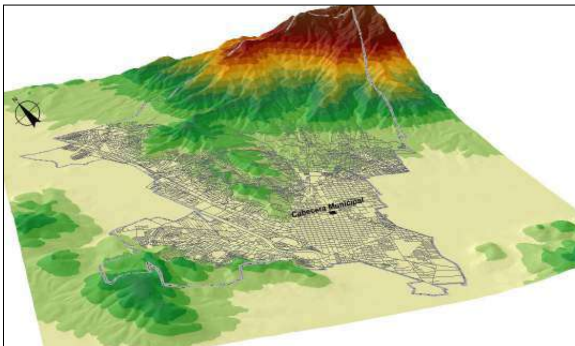
Figura 1.1. Vista en 3D que muestra un modelo del relieve del municipio de Oaxaca de Juárez. Nótese que más de la mitad del área está conformada por una morfología accidentada con elevaciones alineadas en dirección NE-SW.
