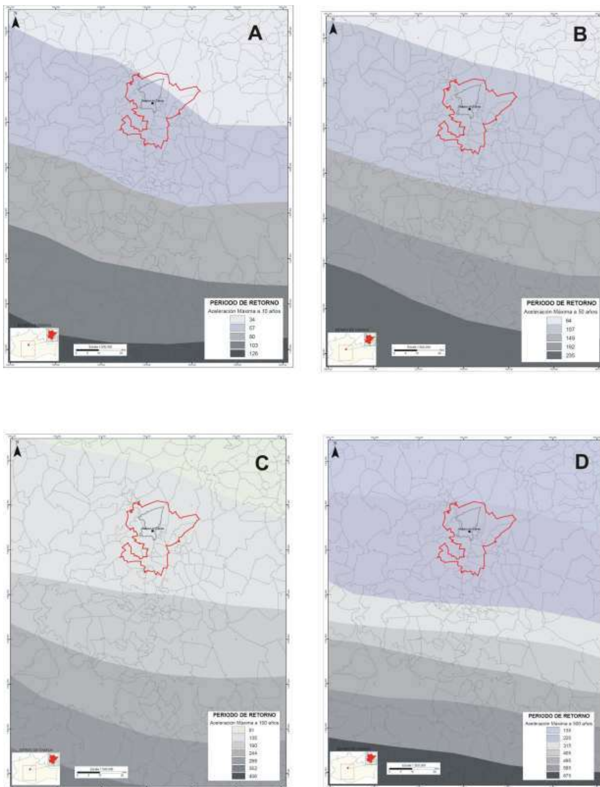
Figura 5.1.4. Mapas de la región central del estado de Oaxaca que muestran diferentes períodos de retorno para aceleraciones máximas A: cada 10 años, B: cada 50 años, C: cada 100 años, D: cada 500 años. Las unidades de las aceleraciones están dadas en gales. Fuente: CENAPRED (2006).
