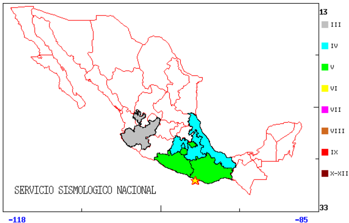
Figura 1.4. Intensidades para el sismo ocurrido en la región de Oaxaca el 14 de junio de 2004 de magnitud 5.8. Fuente: Servicio Sismológico Nacional ( http://www.ssn.unam.mx ).
