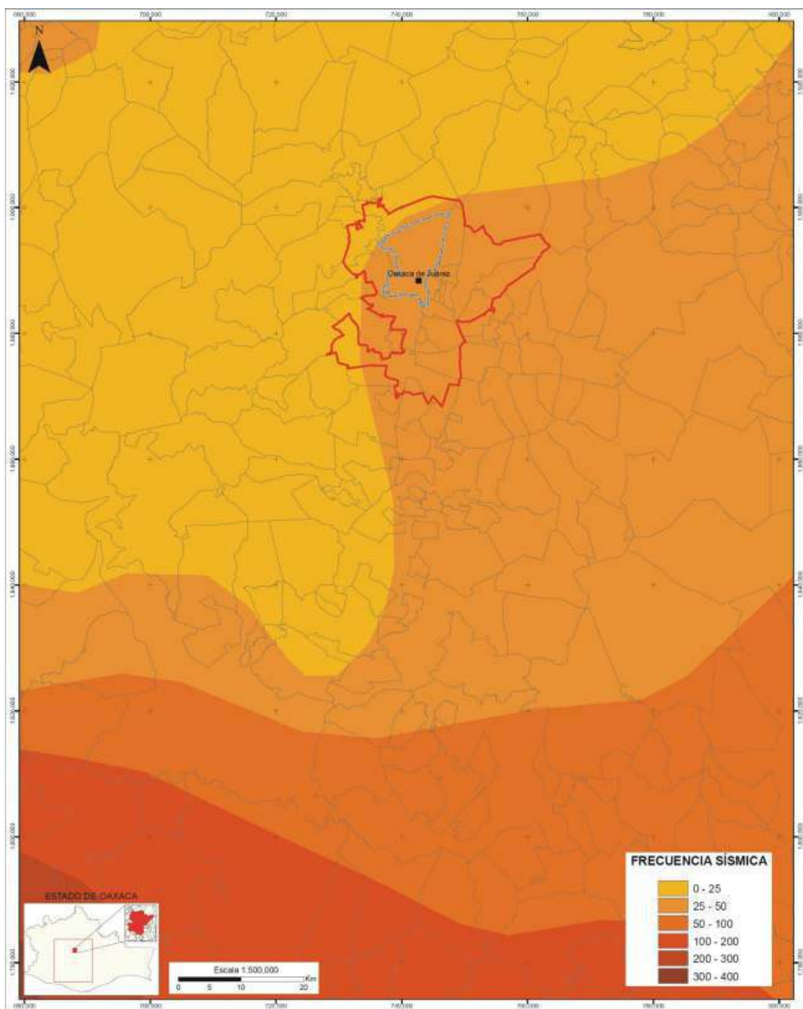
Figura 5.1.3. Mapa de frecuencia sísmica para la región central del estado de Oaxaca entre el período comprendido entre 1998-2011. Fuente: Catálogo de sismos del Servicio Sismológico Nacional período 1998-2011.
