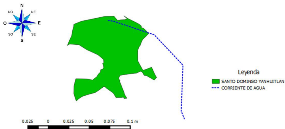
Figura 3. Hidrología
