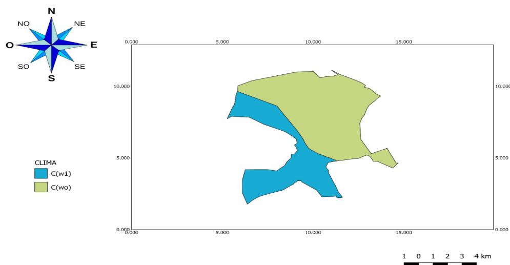
Figura 4. Clima.
