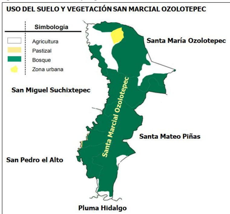
Figura 27. Uso del suelo y vegetación.
