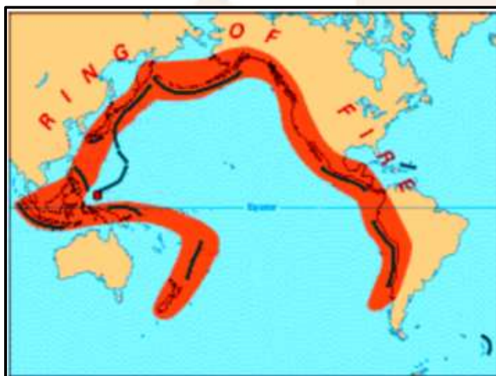
Imagen 3.1. Cinturón circumpacífico
